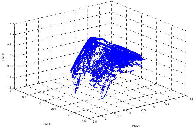
Fig. 5 3-PMD space.
